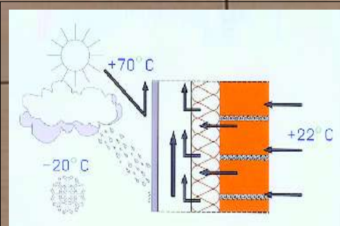
sl.1 Princip ventiliranja fasade
